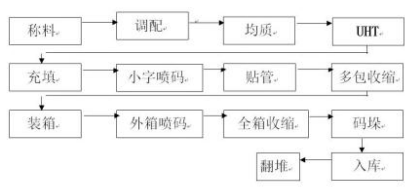
图 3.2 牛奶工艺流程图
