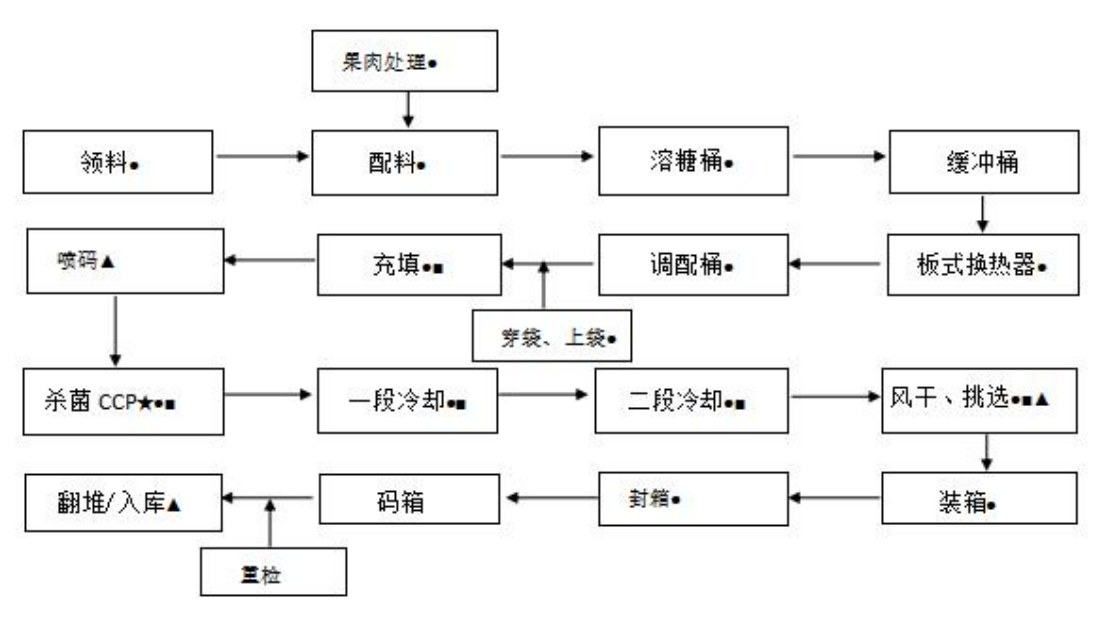
图 3.2 果粒多工艺流程图
