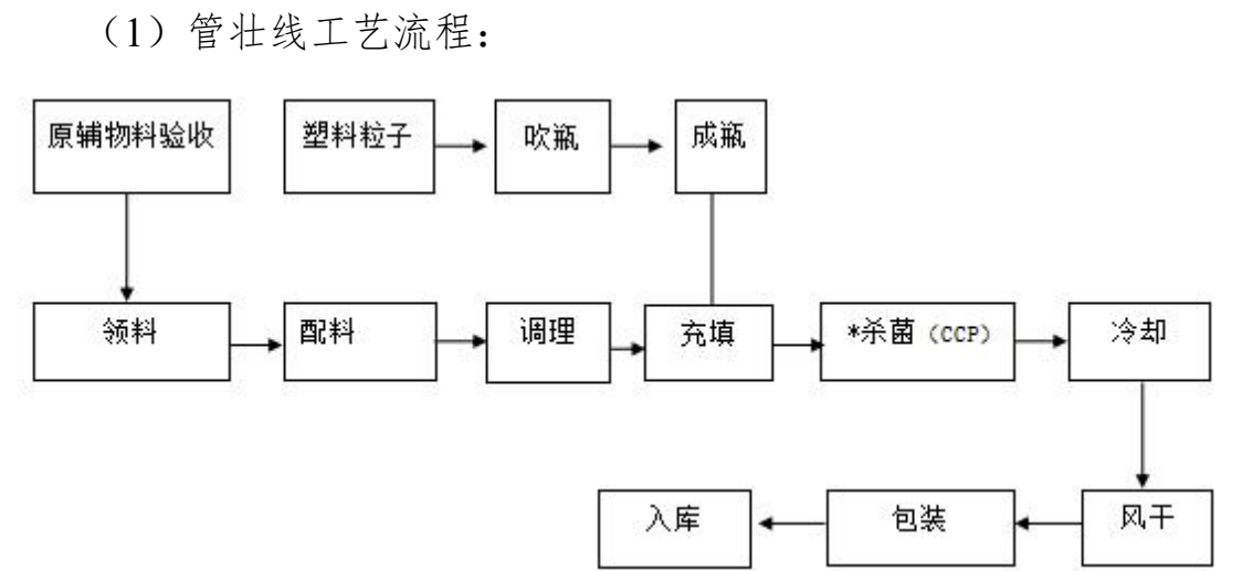
图 3.1 管壮线工艺流程图
